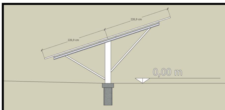
Figura 03 – Estrutura metálica com as placas
