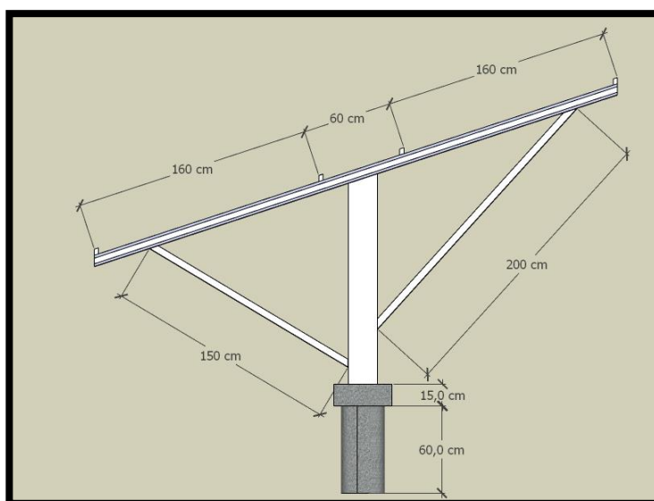
Figura 02 – Estrutura metálica
